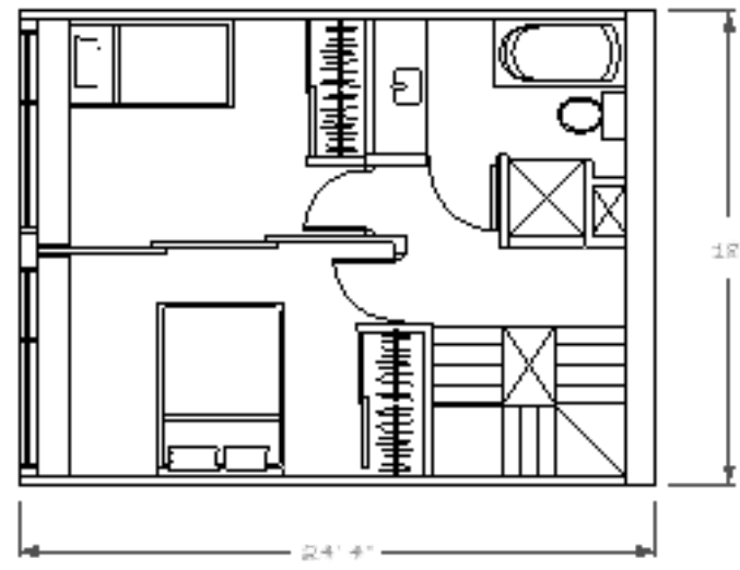
2E ÉTG / 3RD FL
